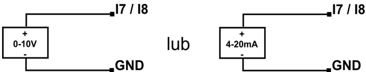
8 Podłączenie źródła napięciowego lub prądowego do wejść skonfigurowanych jako analogowe.
