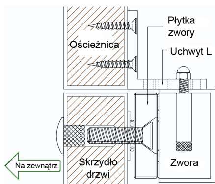
Montaż uchwyty
