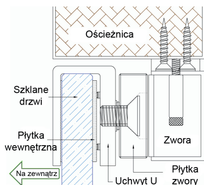
Montaż uchwyty
