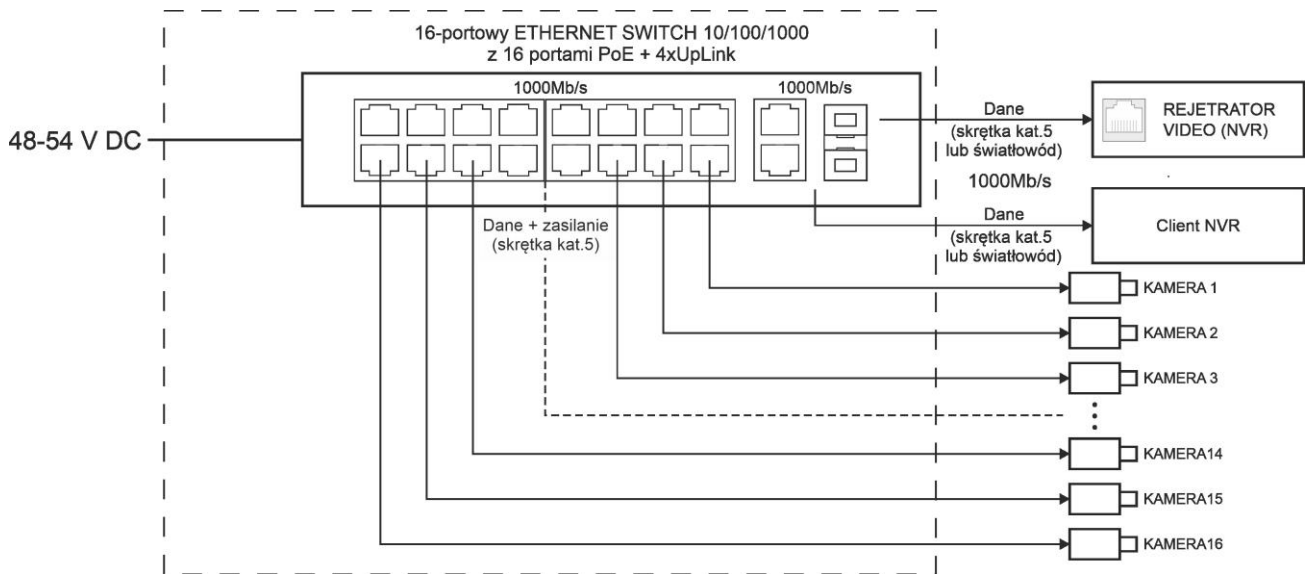
Rys. 1. Schemat blokowy.
