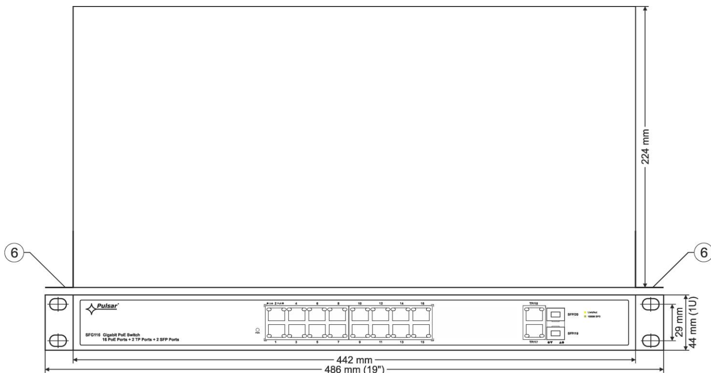
Rys. 4. Widok switch'a.
