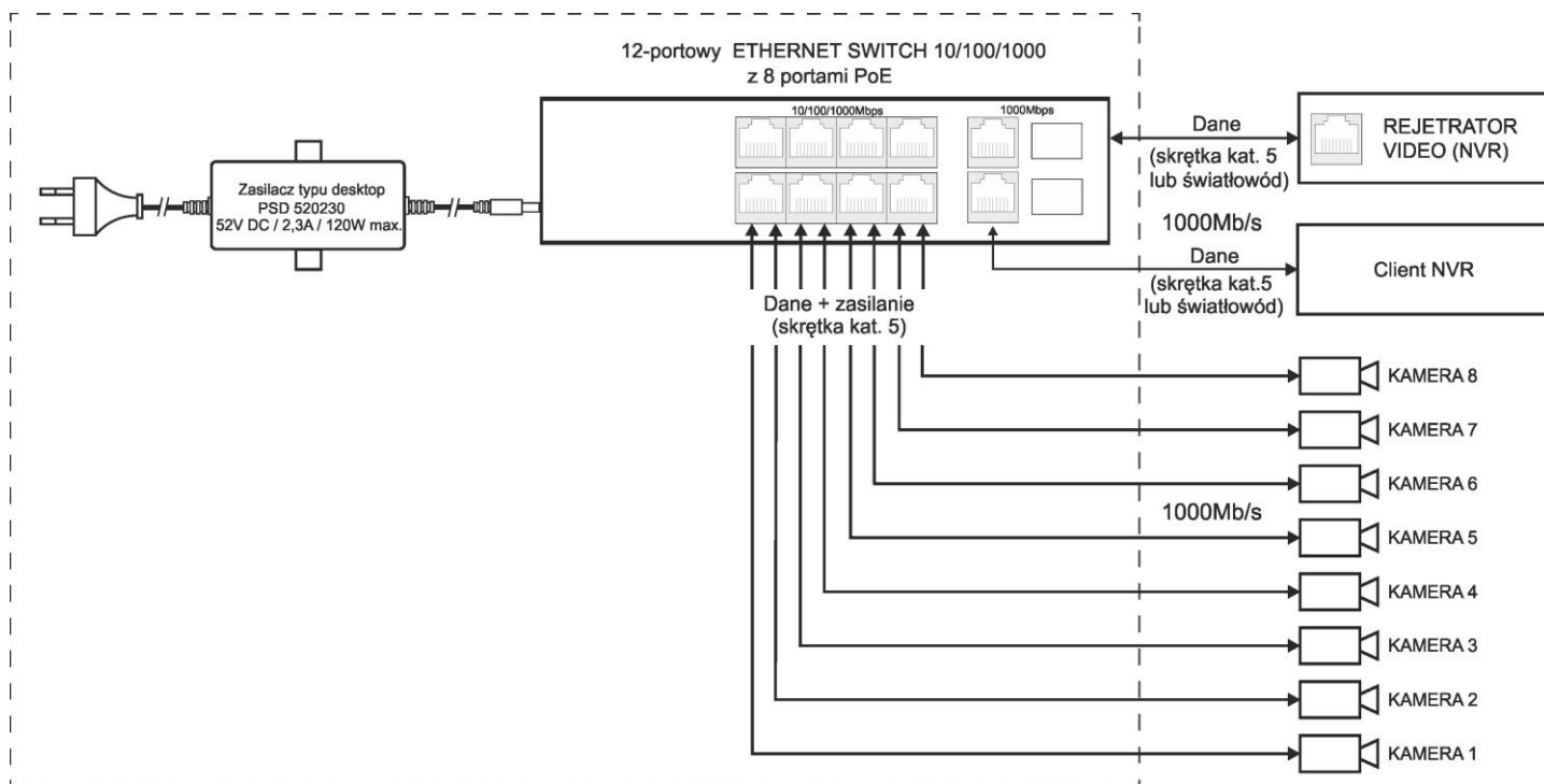
Rys. 1. Schemat blokowy.
