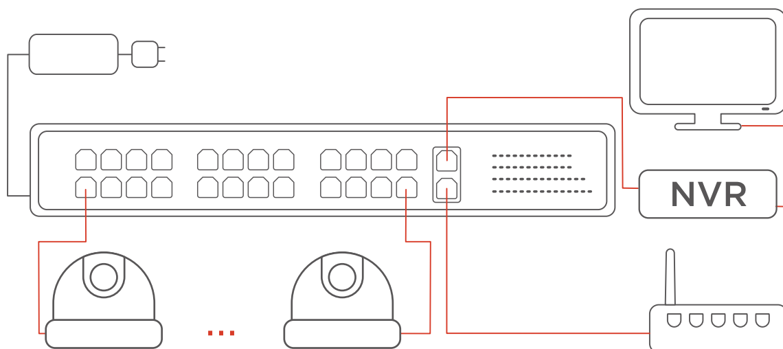
Schemat przykładowego podłączenia PIX-POE24AT-2GE
