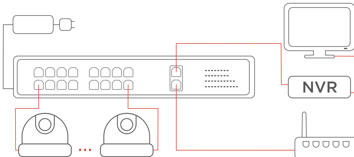
Schemat przykładowego podłączenia PIX-POE16AT-2GE
